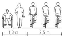
DUBBELRIKTAD GÅNG- OCH CYKELBANA
