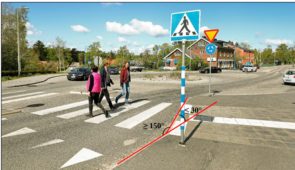
Figur 25 Vinklar mot en körbana ska inte göras snävare än 150°
