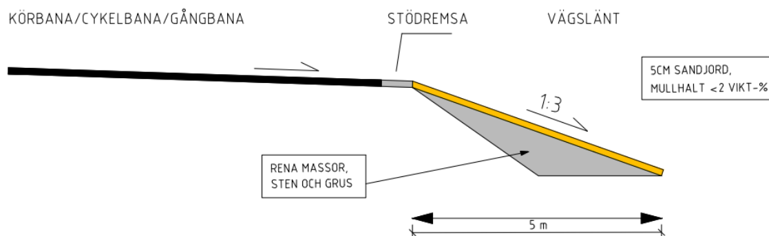
Figur 14 Principskiss för anläggning av väglänt. Mager jord ska användas, med en mullhalt lägre än 2 viktprocent. Observera att insädd av frön ska undvikas, i första hand ska befintlig förna tas tillvara och återanvändas.
