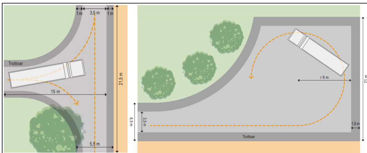
Figur 18 Minsta mått för vändning med avfallsfordon, med respektive utan backning. Med annan form på vändplatsen behöver måtten utökas. Illustration av Sara Sundin, Ramboll, hämtad från Avfall Sveriges publikation Handbok för avfallsutrymmen.
