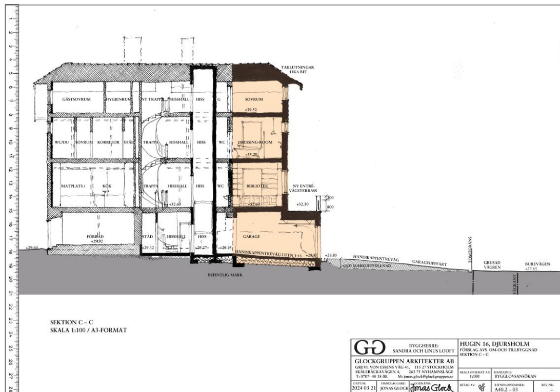
Figur 3: Sektion som visar tänkt tillbyggnad mot Burevägen. Framtagen av Glockgruppen Arkitekter AB.
