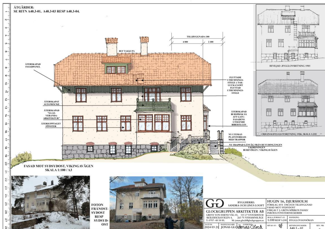
Figur 5: Fasad efter tillbyggnad, sedd från Vikingavägen. Framtagen av Glockgruppen Arkitekter AB.
