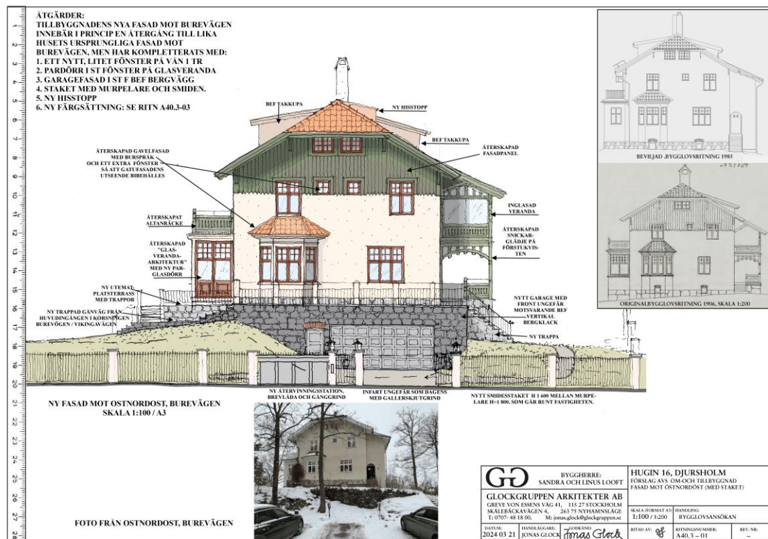
Figur 4: Fasad efter tillbyggnad sedd från Burevägen. Framtagen av Glockgruppen Arkitekter AB.
