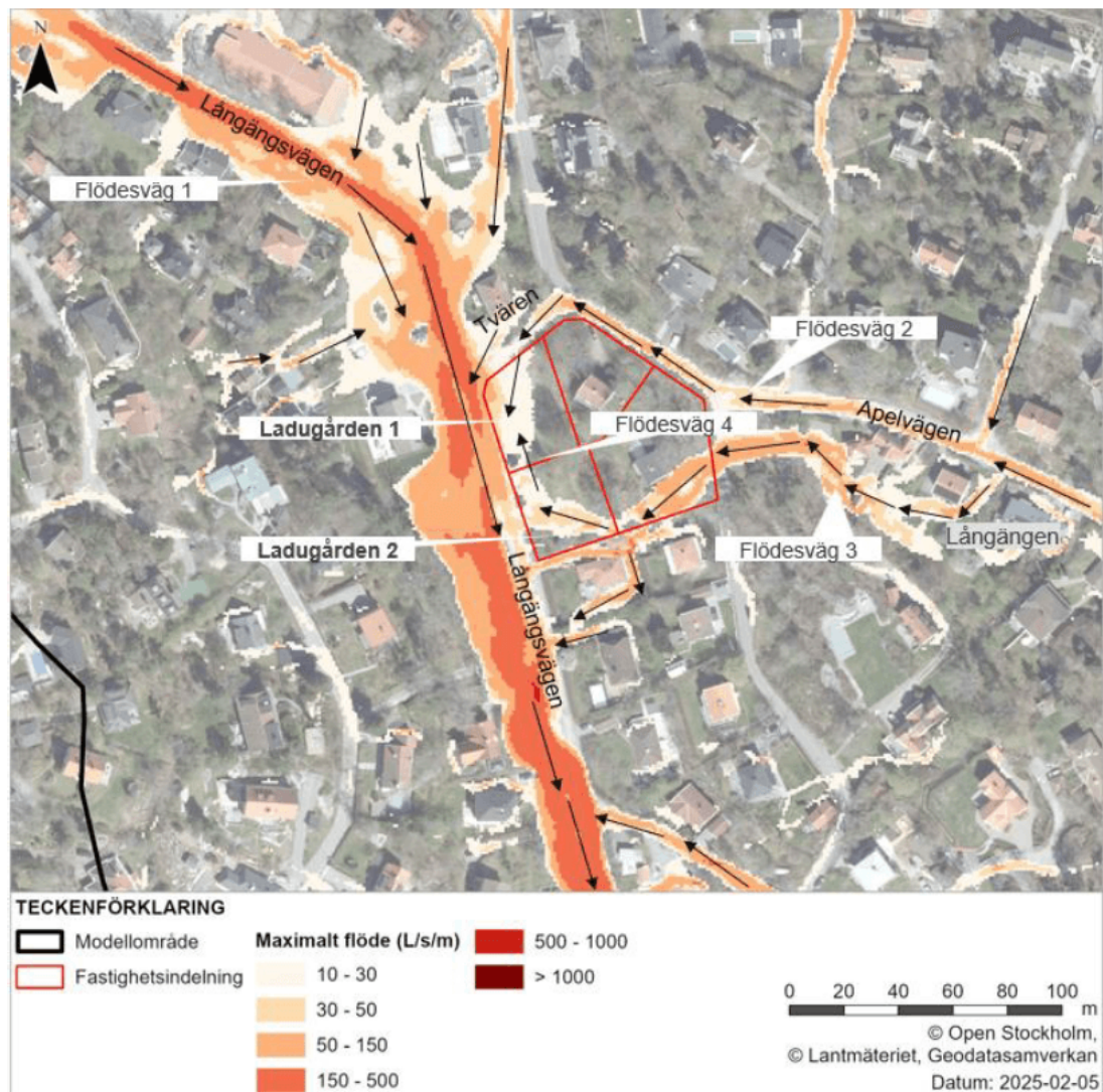
Figur 11: Flödesvägar och maximalt flöde inom och runtom planområdet enligt framtagna utredning (Sweco 2025).
