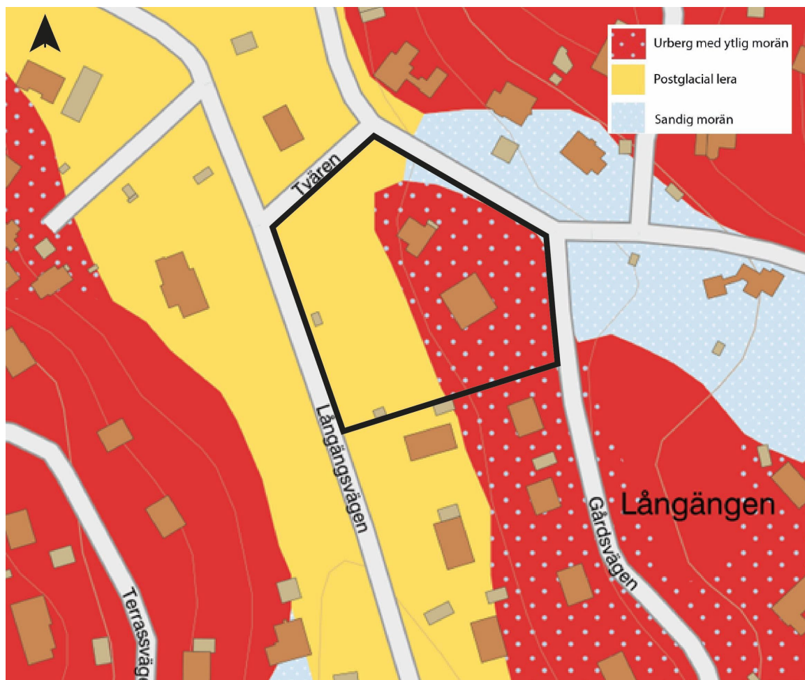
Figur 10: Jordarter inom planområdet (SGU).
