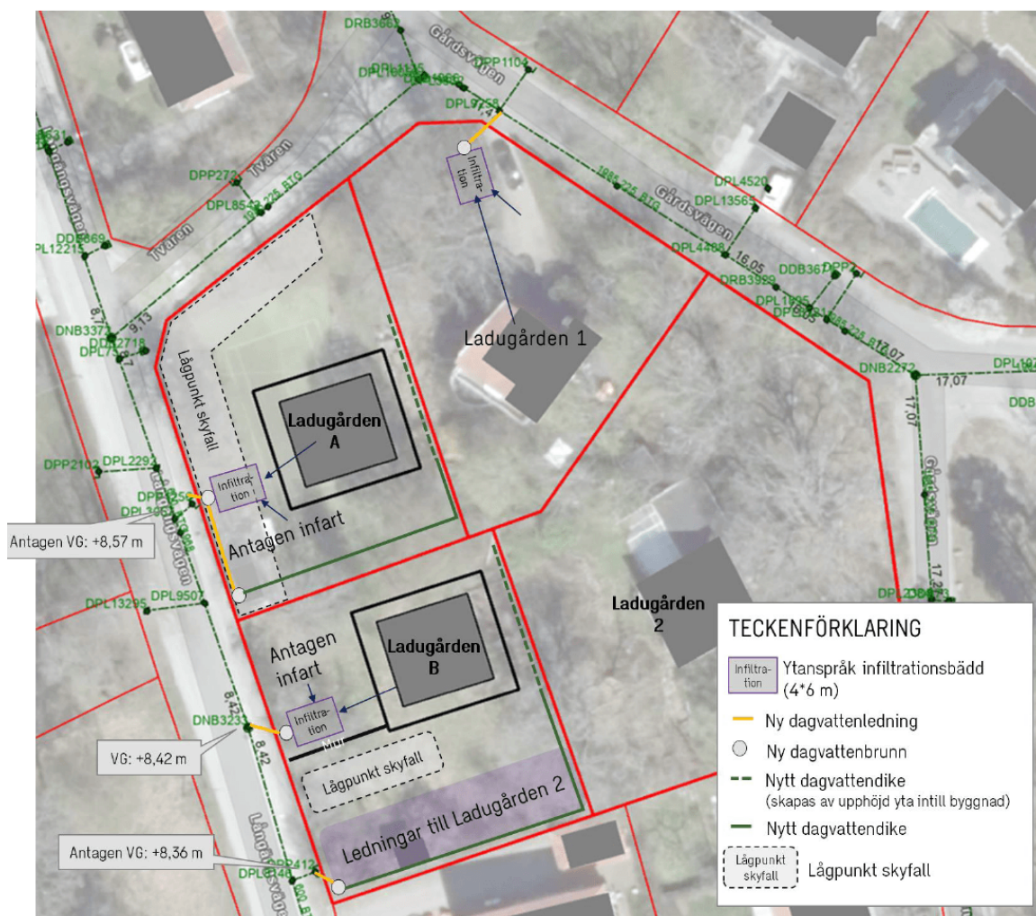
Figur 9: Föreslagna dagvatten samt skyfallslösningar inom de avstyckade fastigheterna (Sweco 2025)
