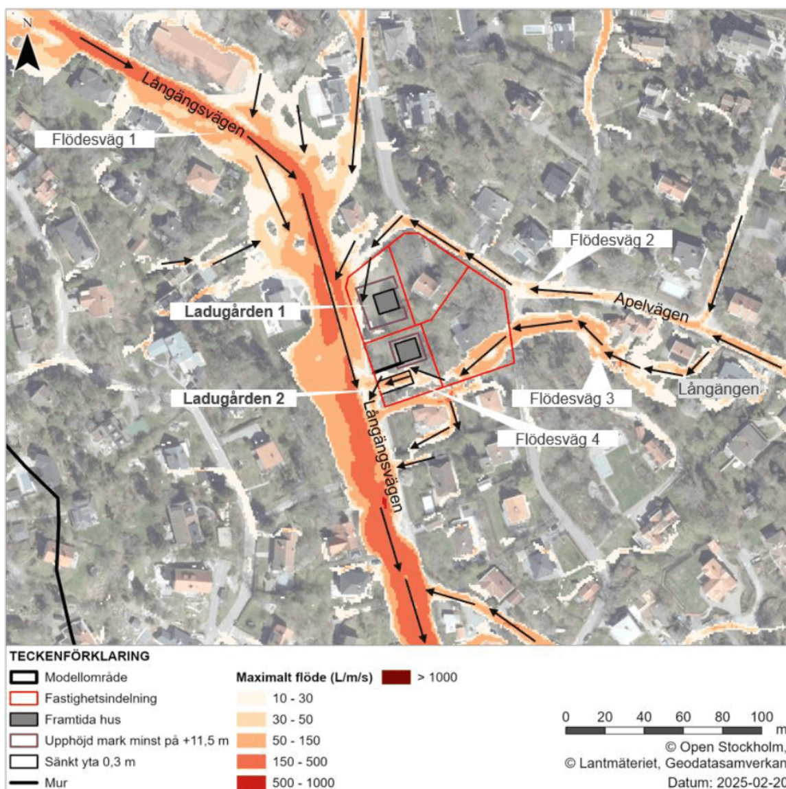
Figur 12: Planförslagets åtgärder för skyfallshantering enligt framtagna skyfallsutredning (Sweco 2025).
