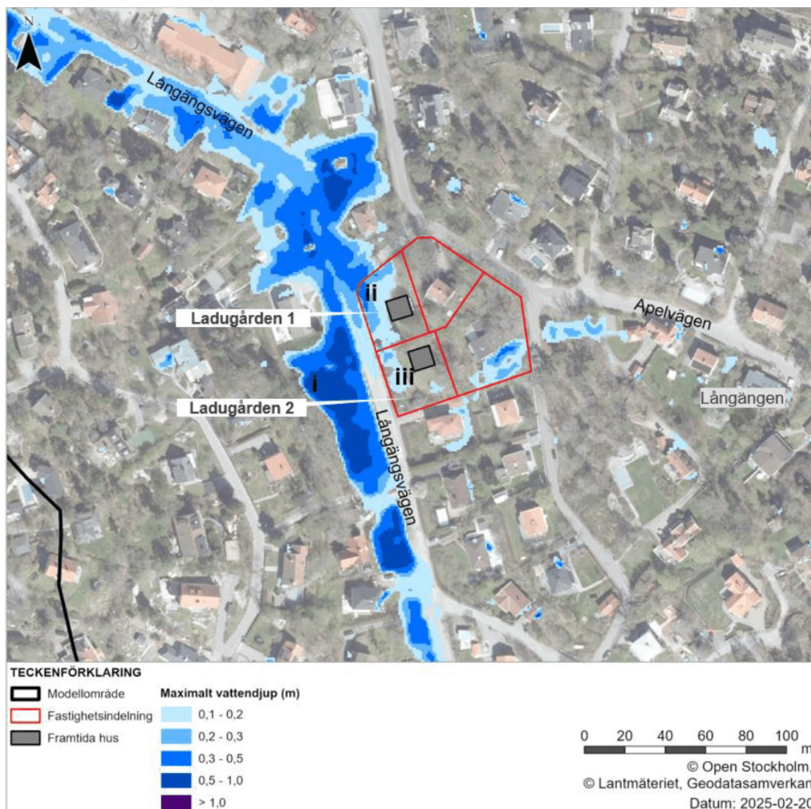
Figur 7: Maxdjup inom och runt planområdet enligt framtagna skyfallsutredning (Sweco 2025).
