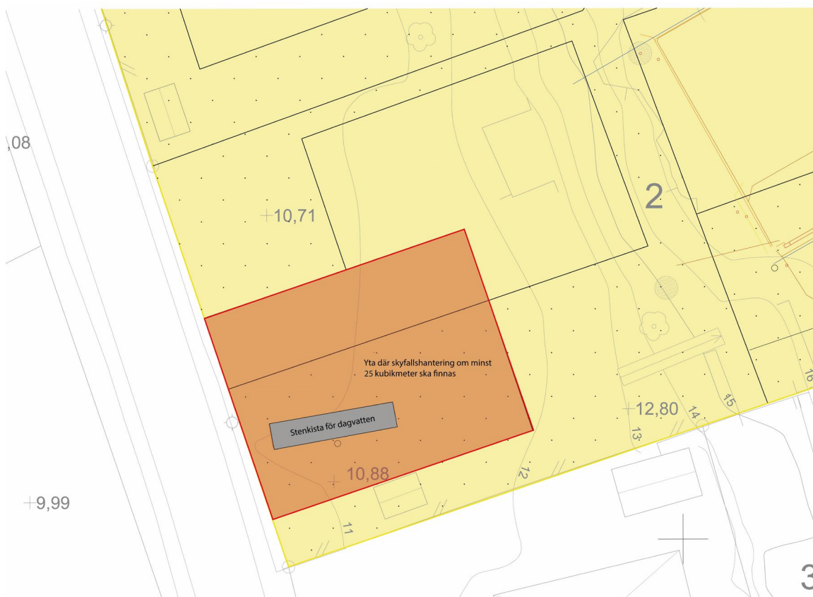
Figur 13: Placering av stenkista och reglerad yta för skyfallshantering inom Ladugården B.
